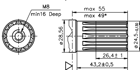
SA - splined, B25x22xH9 DIN 5482 Max. Torque 40 daNm
